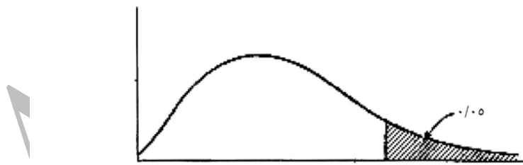
شکل ۱ سطح زیر منحنی H_0 و H_1 با \alpha = 0/05
